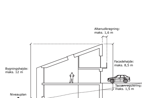
Principsnit af rækkehusbebyggelse i byggefelt B.
