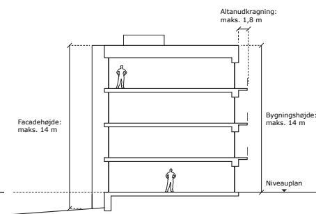
Principsnit af etageejendom i byggefelt A1
