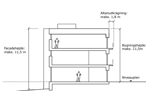
Principsnit af etageejendom i byggefelt A2
