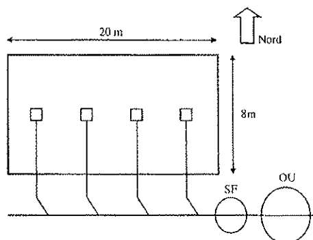
Figur 4.4 Overdækket salgsplads med 4 nedløbsbrønde
