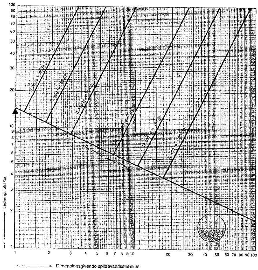
Figur 4.6 Dimensioneringsdiagram for udluftede spildevandsledninger af plast- og rustfrit stål
